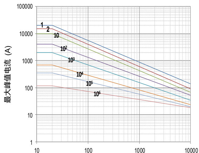
脉冲持续时间 (μs) SFV34S470K to SFV34S680K
